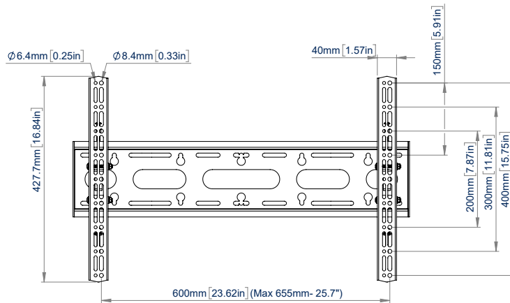
VOORAANZICHT
