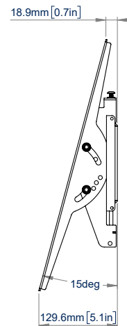
ZIJAANZICHT MAXIMALE KANTELHOEK
