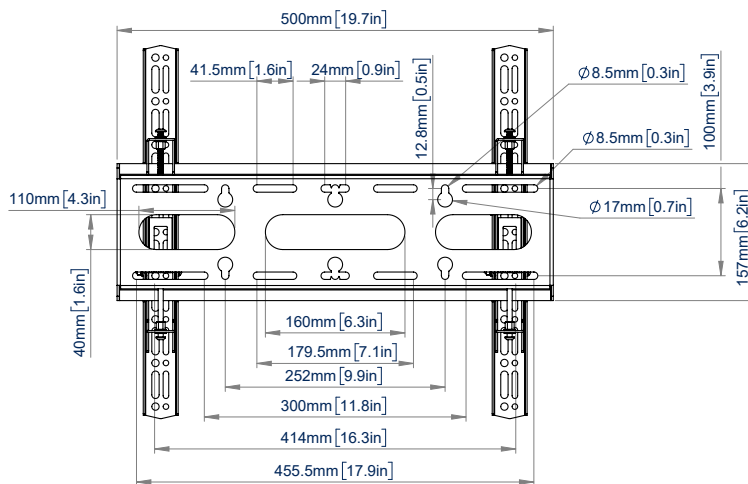
ACHTERKANT
