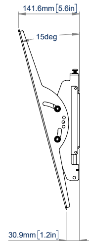
ZIJAANZICHT MAXIMALE KANTELHOEK
