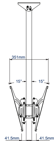
ZIJAANZICHT INTERFACE NAAR BENEDEN KANTELEN
