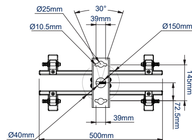
BOVENAANZICHT
