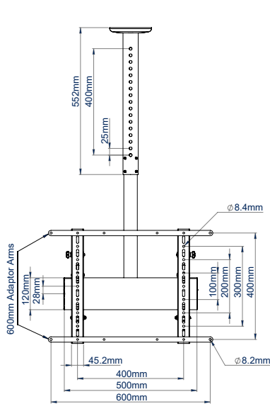
VOORAANZICHT
