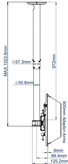
ZIJAANZICHT MAXIMALE VERLENGING
