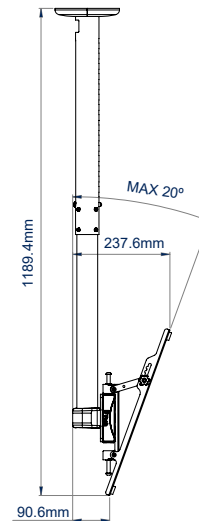
ZIJAANZICHT MET KANTELING
