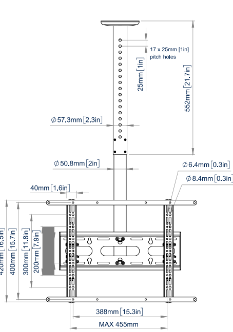
VOORAANZICHT
