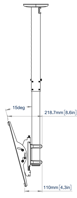
ZIJAAANZICHT MET KANTELFUNCTIE
