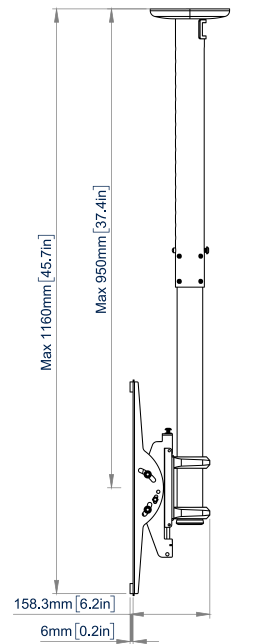
ZIJAAANZICHT MAXIMALE VERLENGING
