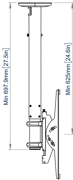
ZIJAAANZICHT MIN UITBREIDING
