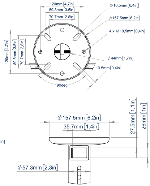
BOVENAANZICHT
