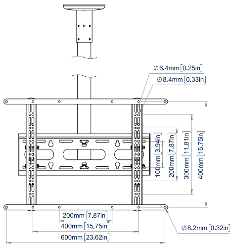
VOORAANZICHT
