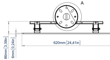
BOVENAANZICHT PLAFONDBEVESTIGING
