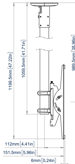
ZIJAANZICHT NEE KANTELING
