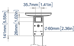
VOORAANZICHT
