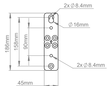
MUURBEUGEL
