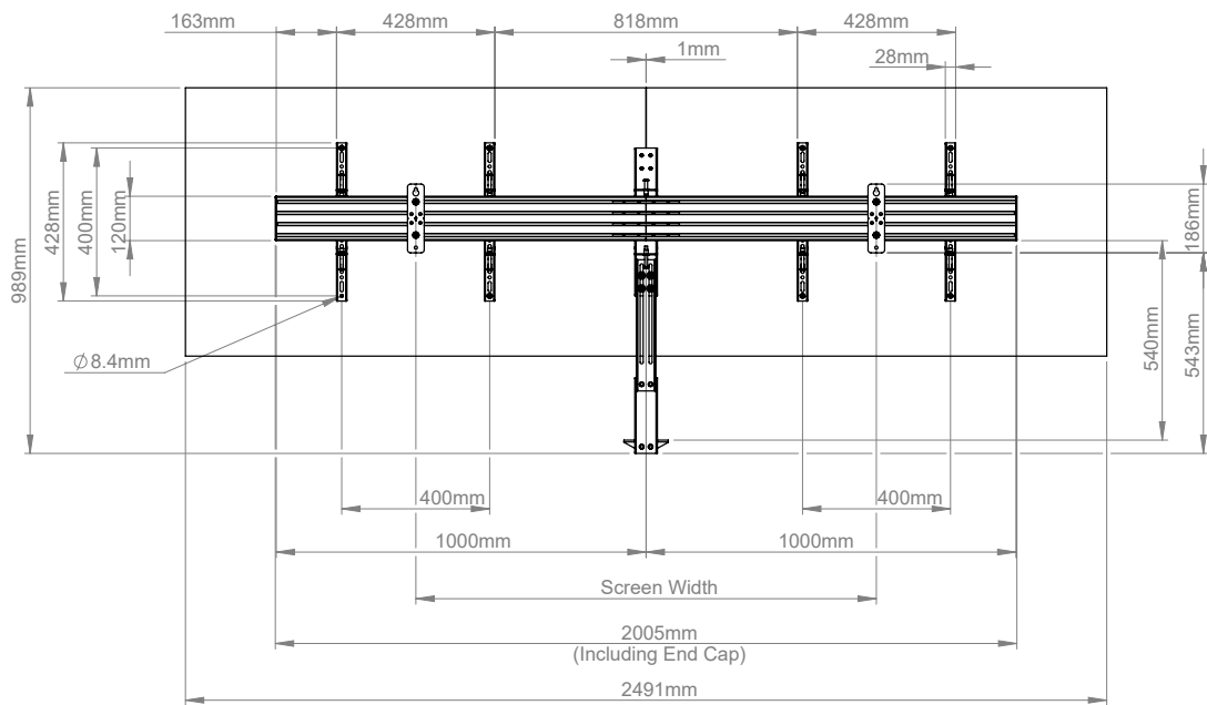
VOORAANZICHT
