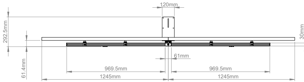
BOVENAANZICHT
