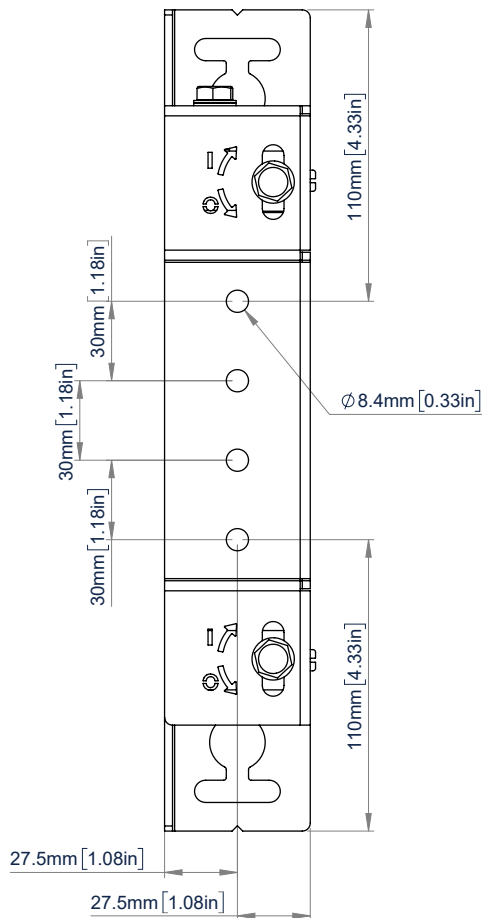
VOORAANZICHT
