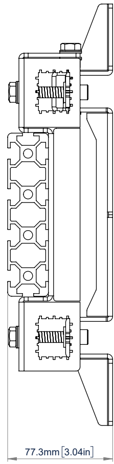
ZIJAANZICHT MET BT8390 MONTAGERAIL MAXIMALE DIEPTE
