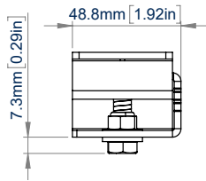
BOVENAANZICHT
