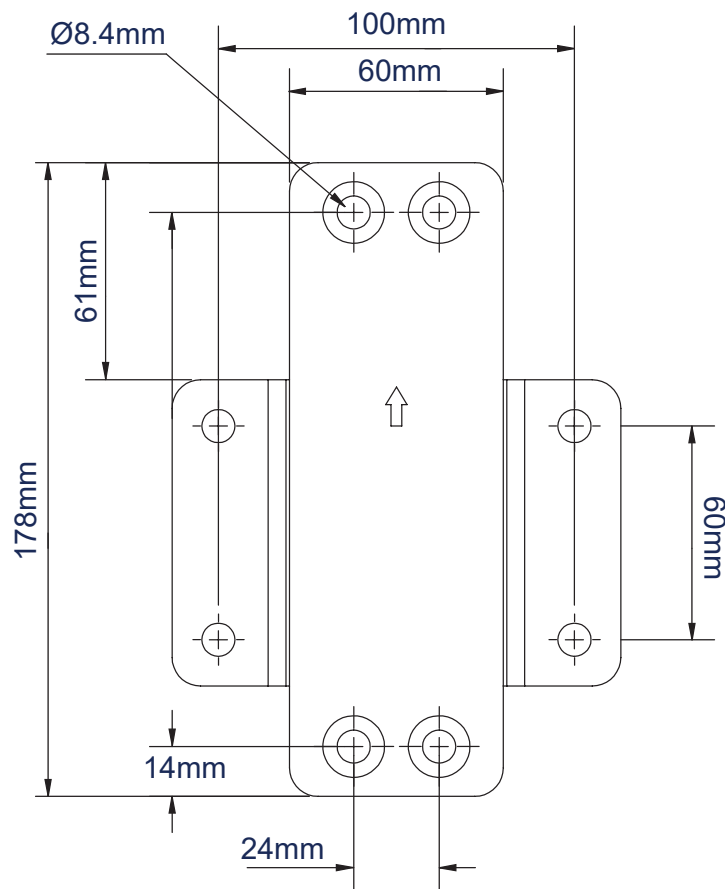
VOORAANZICHT
