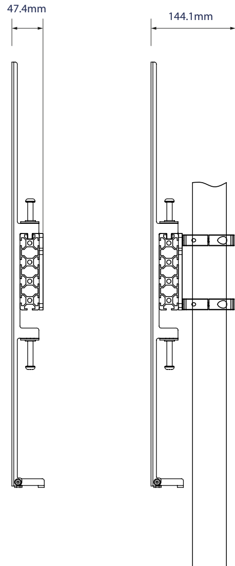
WANDMONTAGE MEER DAN 1 RAIL*
