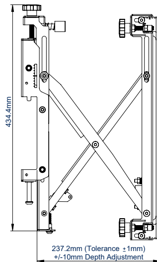
ZIJAANZICHT - UITGEBREID
