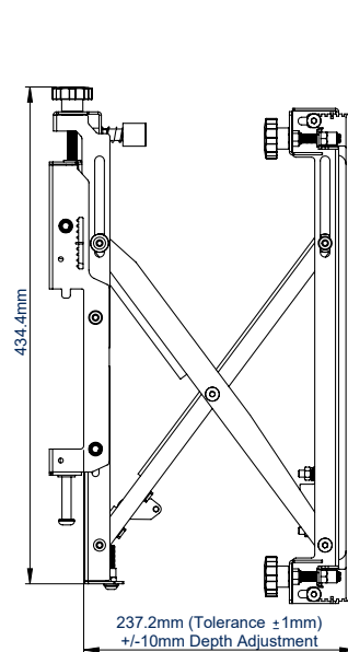
VISTA LATERAL - AMPLIADA
