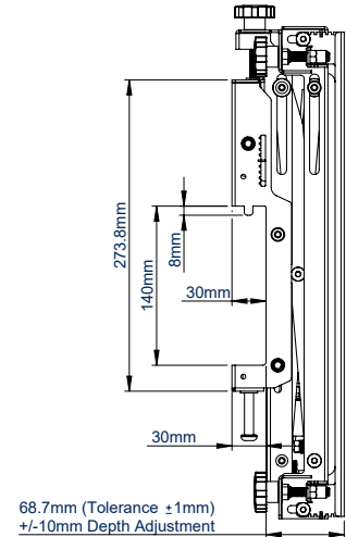
VISTA LATERAL - CERRADO
