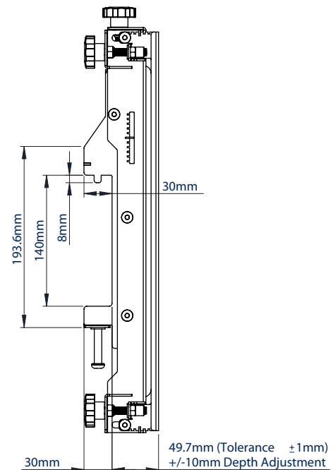
ZIJAANZICHT
