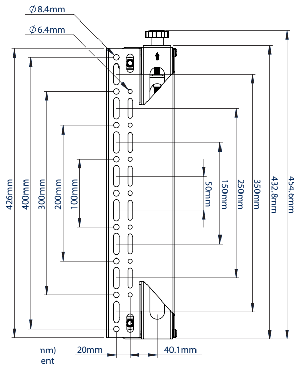
VOORAANZICHT
