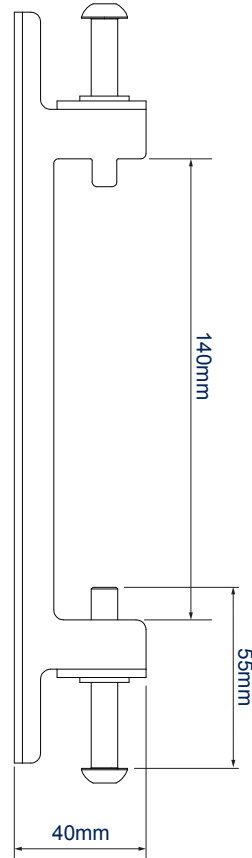
ZIJAANZICHT
