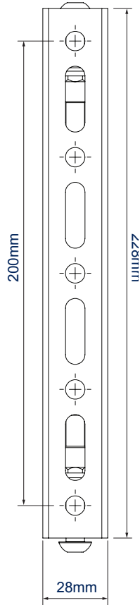
VOORAANZICHT
