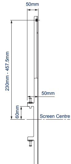
ZIJAANZICHT BOVEN DE RAIL
