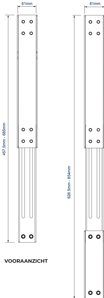
VOORAANZICHT MET VERLENGSTANG
