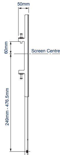
ZIJAANZICHT ONDER DE RAIL
