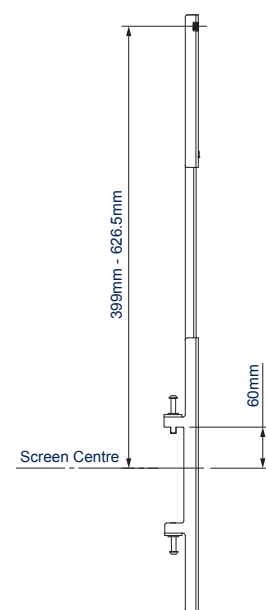
ZIJAANZICHT MET VERLENGSTANG BOVEN DE RAIL
