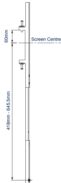
ZIJAANZICHT MET VERLENGSTANG ONDER DE RAIL
