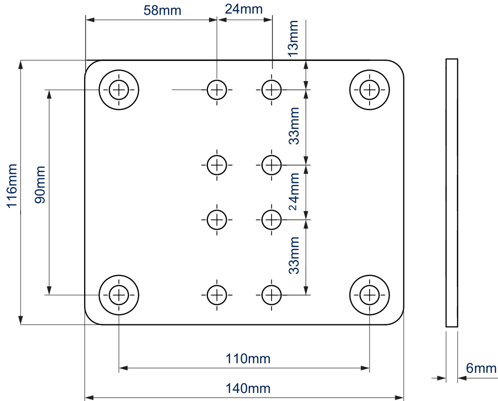
VOORAANZICHT
