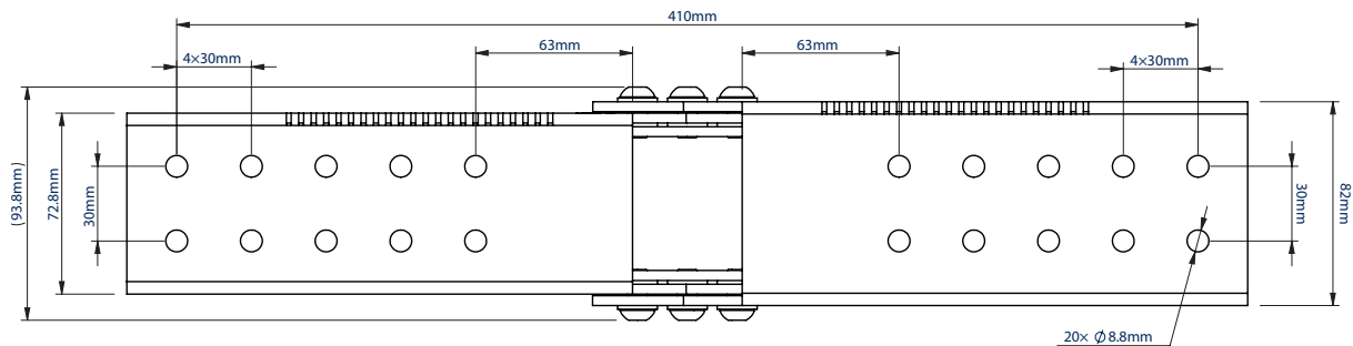
VOORAANZICHT
