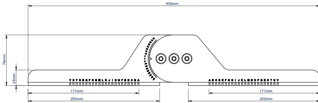
VOORAANZICHT
