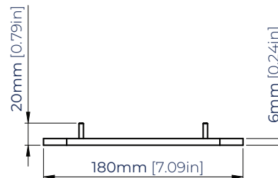
VOORAANZICHT
