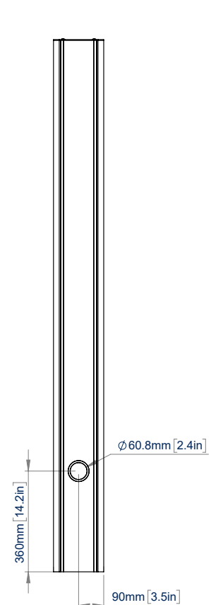
ACHTERAANZICHT
