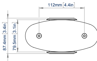
BOVENAANZICHT
