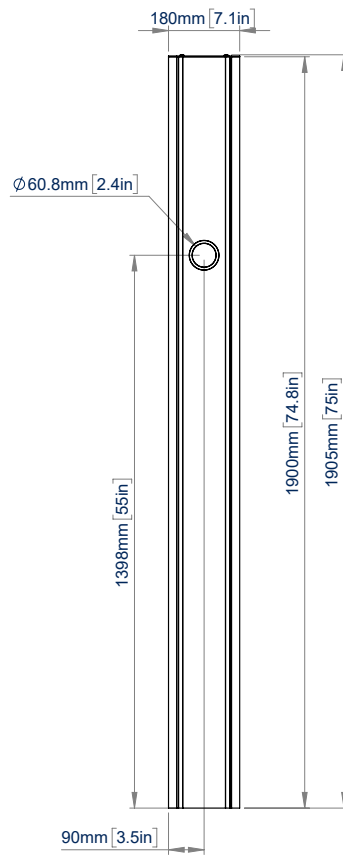
BT8385-190 VOORAANZICHT
