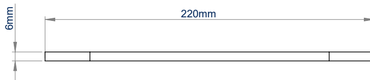
VOORAANZICHT
