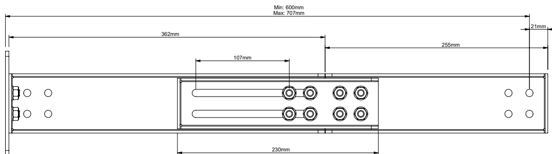
ZIJAAANZICHT - VERBINDINGSPLAAT MET LANGE VERLENGPLAAT
