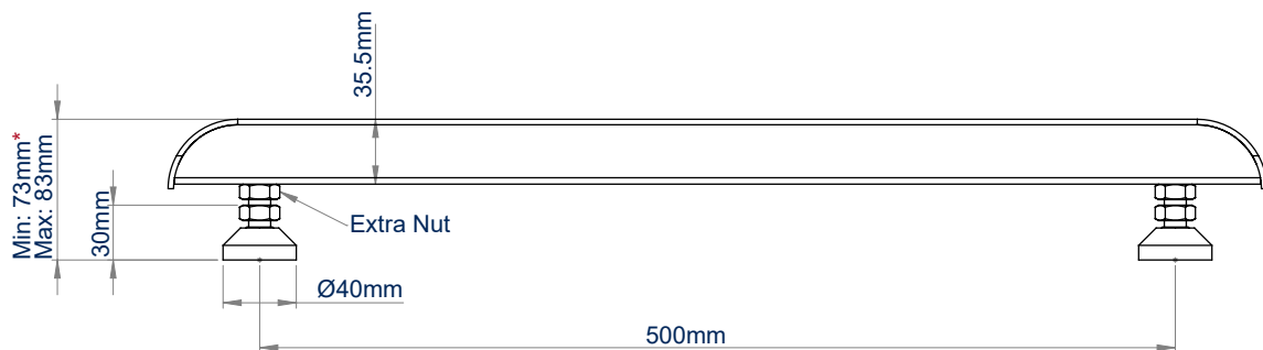
ZIJAAANZICHT
