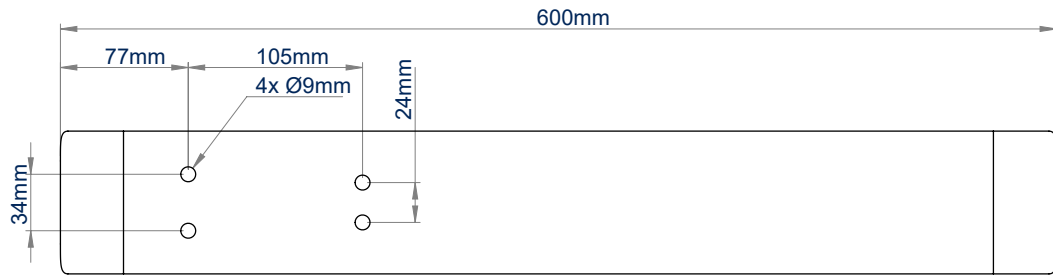
BOVENAANZICHT
