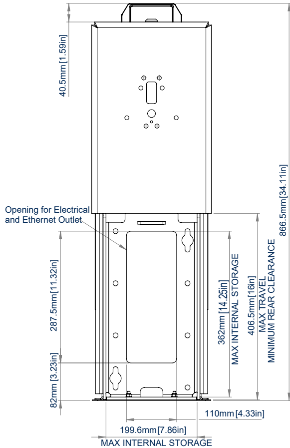
BOVENAANZICHT OPEN
