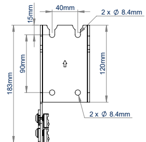
VOORAANZICHT
