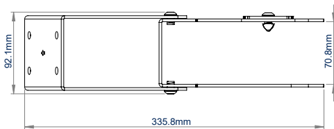
BOVENAANZICHT
