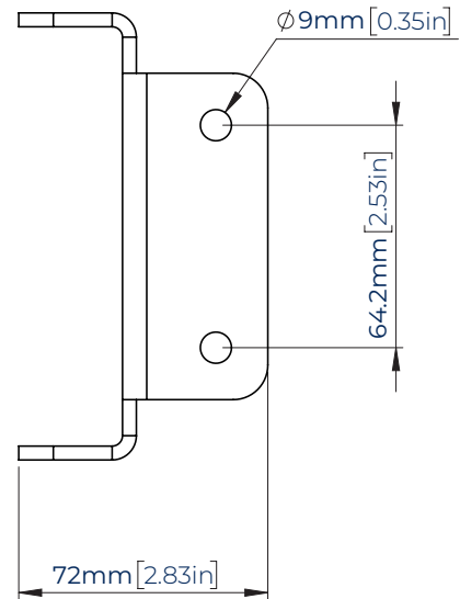
ZIJAANZICHT
