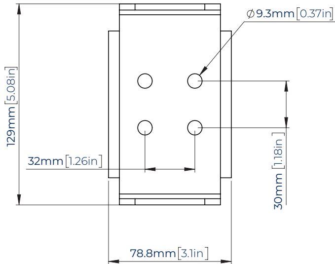
VOORAANZICHT
