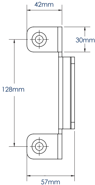
ZIJAAANZICHT
