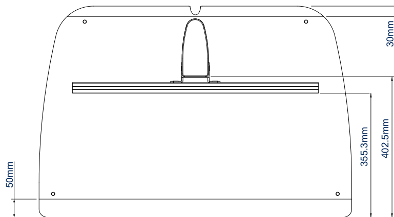
BOVENAANZICHT MET BT8380, BT8380-JPK & BT8390-050
