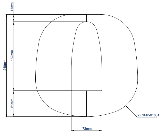
VOORAANZICHT
