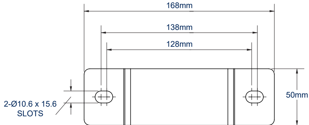
BOVENAANZICHT
