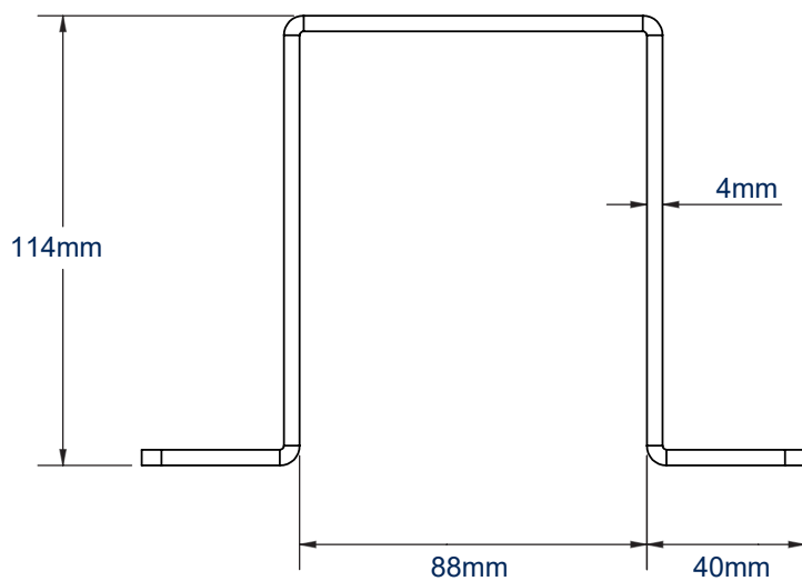
ZIJAANZICHT
