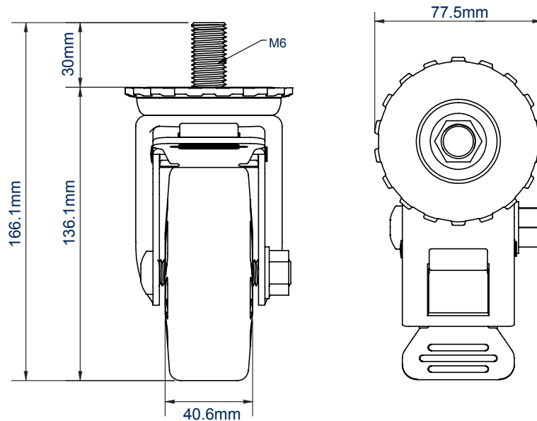
VOORAANZICHT
