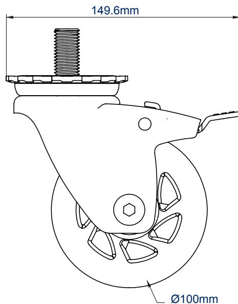
ZIJAANZICHT
