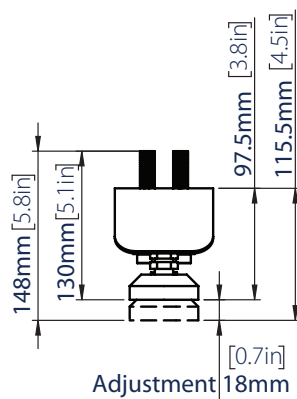
VOORAANZICHT
