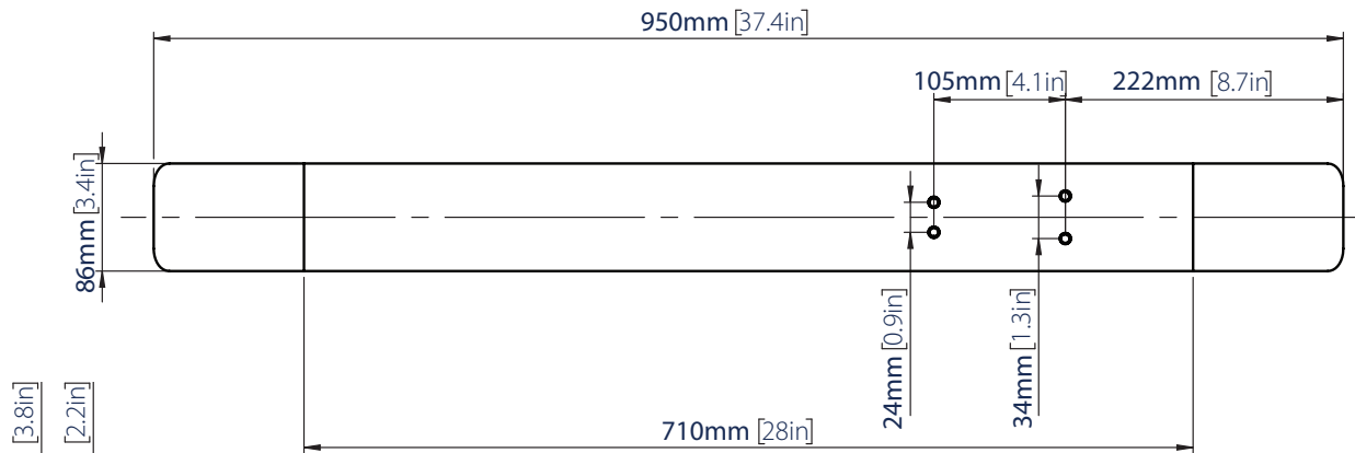
ZIJAAANZICHT
