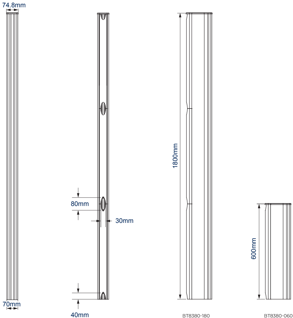
VOORAANZICHT
