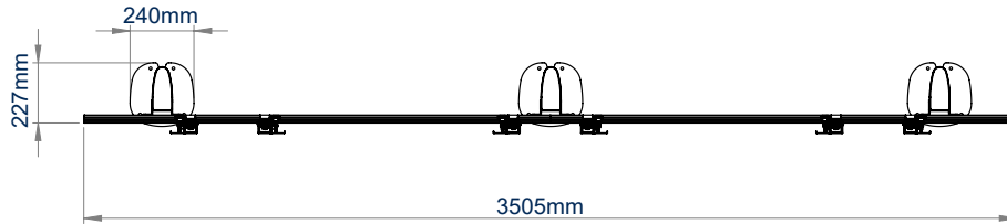
BOVENAANZICHT
