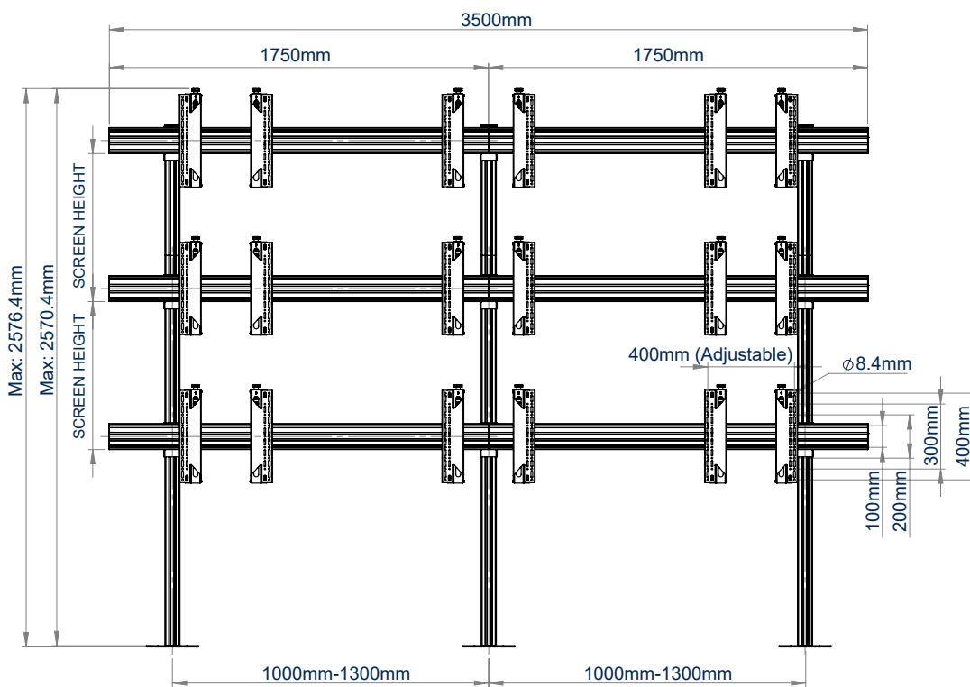
VOORAANZICHT
