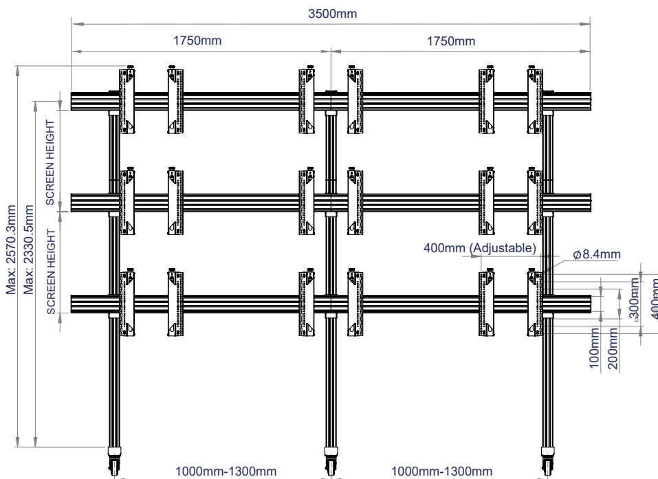
VOORAANZICHT
