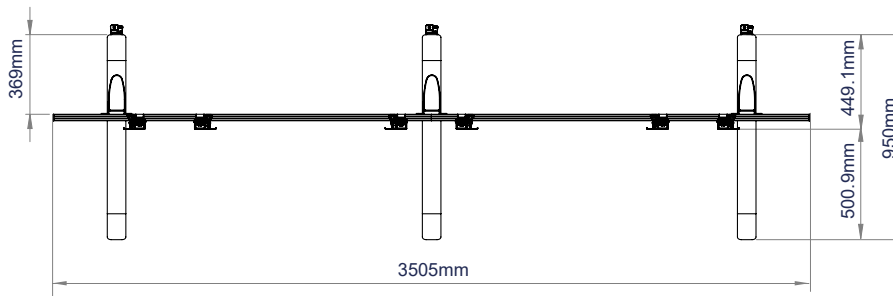
BOVENAANZICHT
