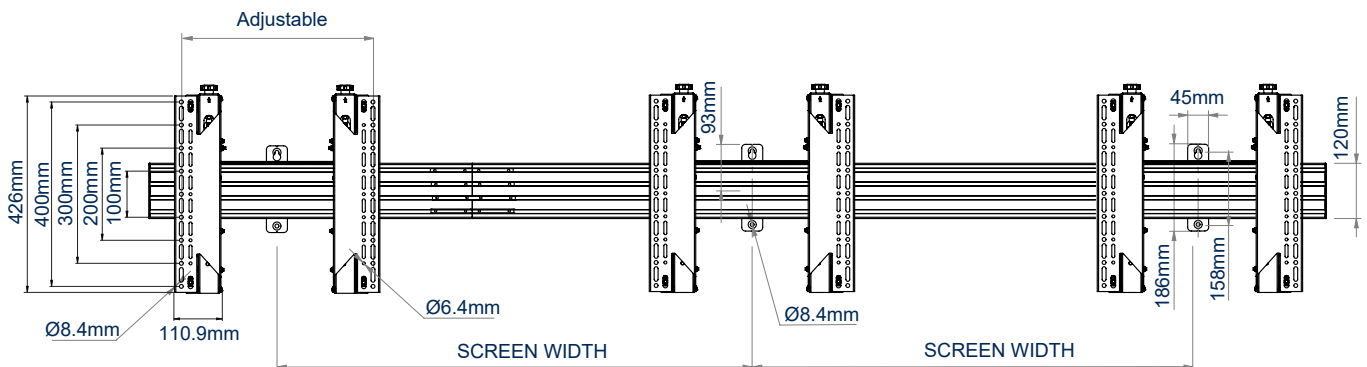
VOORAANZICHT
