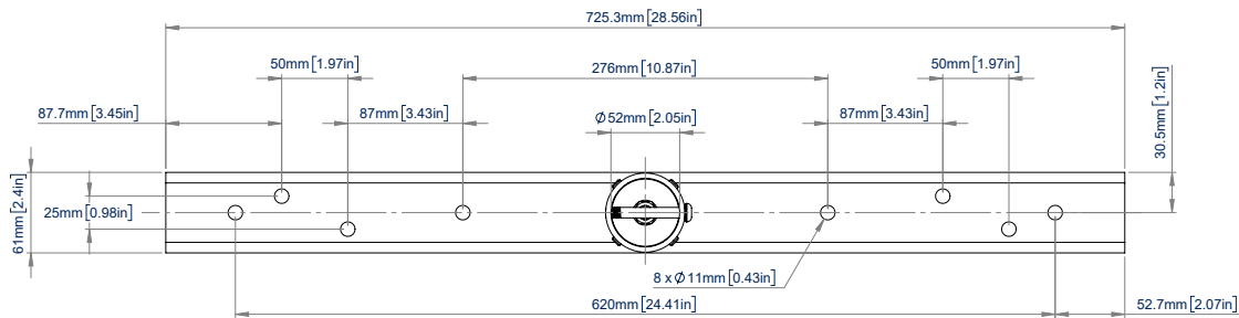
BOVENAANZICHT
