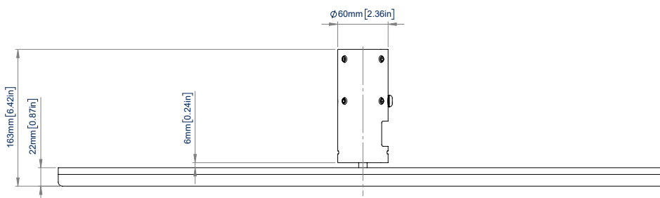
VOORAANZICHT
