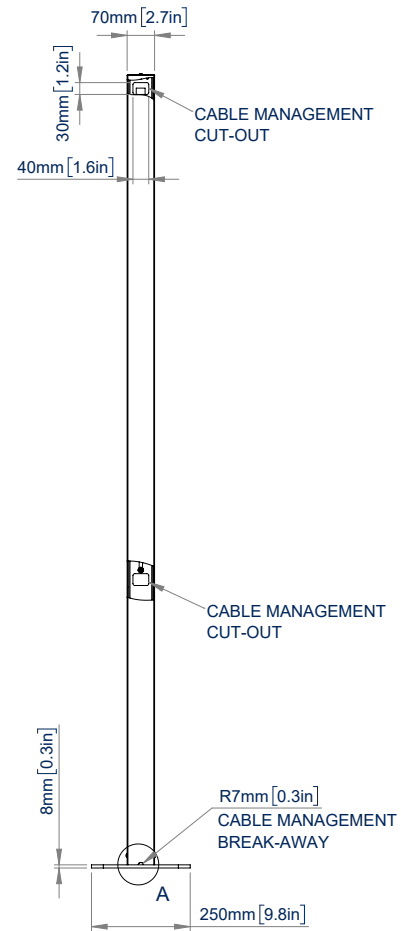
ZIJAANZICHT
