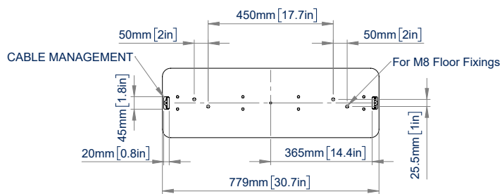
BOVENAANZICHT
