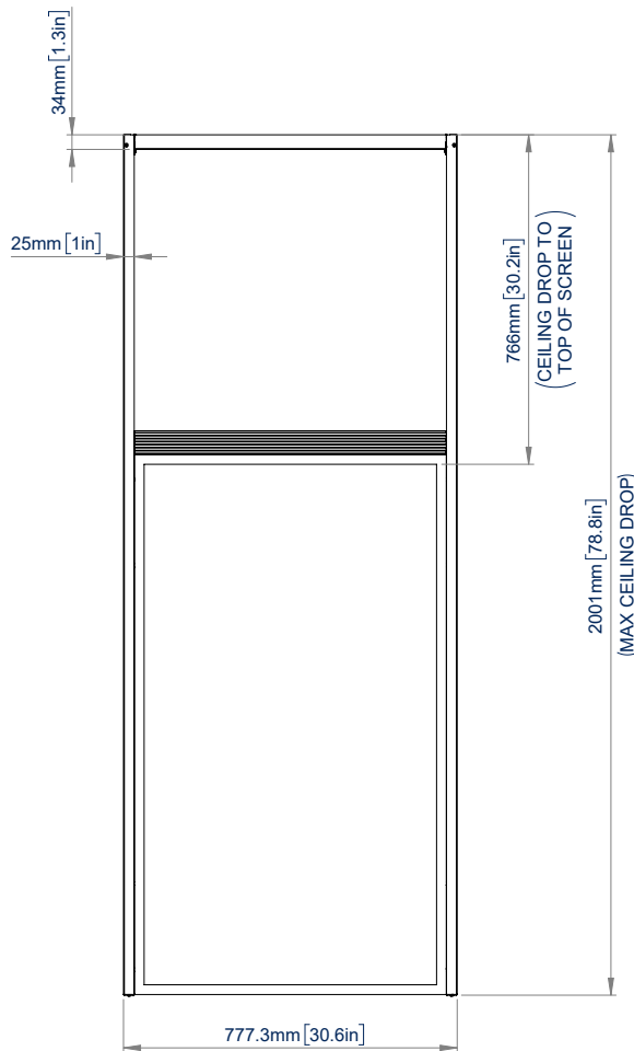
VOORAANZICHT
