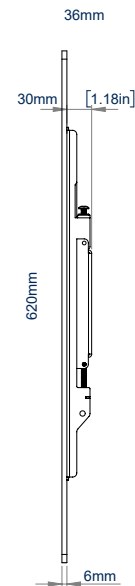
ZIJAANZICHT
