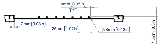
BOVENAANZICHT
