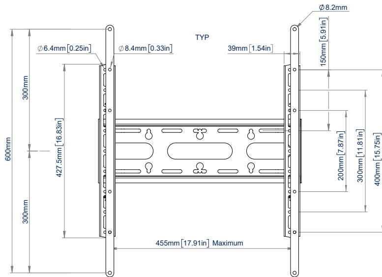
VOORAANZICHT
