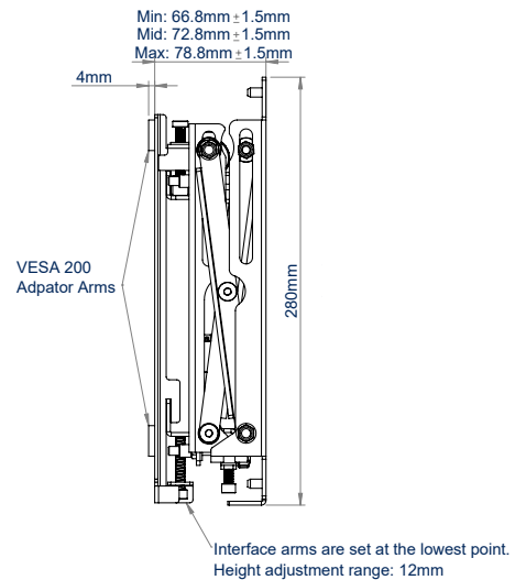
ZIJAANZICHT GESLOTEN
