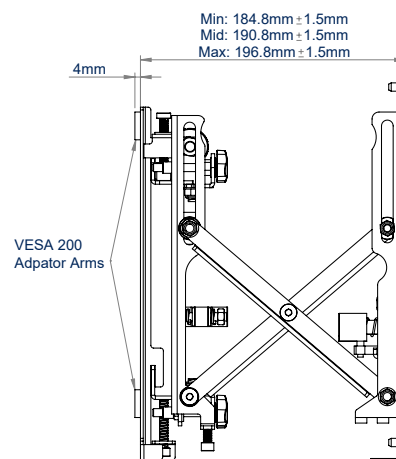
ZIJAANZICHT UITGEBREID
