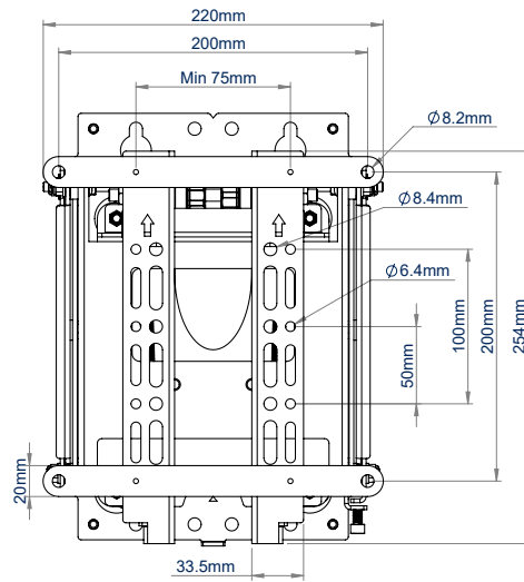
VOORAANZICHT MET ADAPTERARMEN
