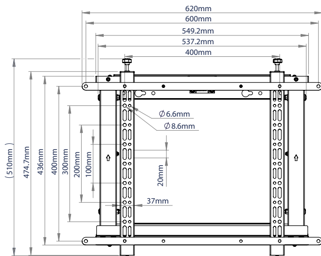
VOORAANZICHT
