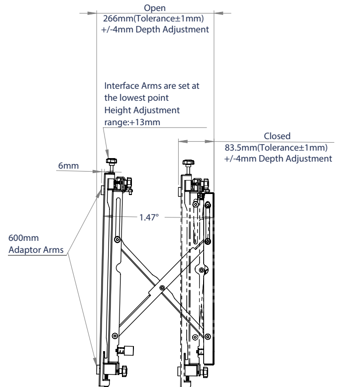
ZIJAANZICHT UITGEBREID
