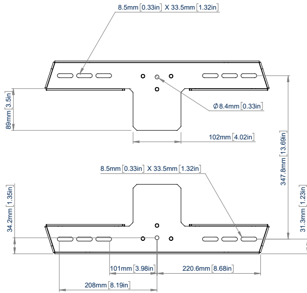
VOORAANZICHT
