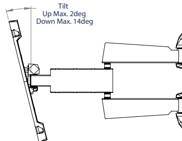
ZIJAANZICHT MAXIMALE UITREKKING
