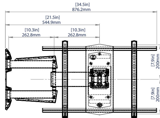
VOORAANZICHT MET ARM UITGEBREID NAAR DE ZIJKANT
