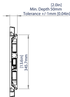
ZIJAANZICHT - VLAK TEGEN DE MUUR
