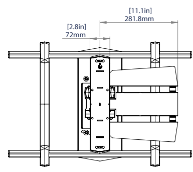
ACHTERAANZICHT
