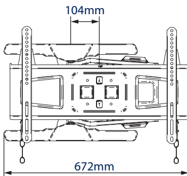
VOORAANZICHT VLAK TEGEN DE MUUR
