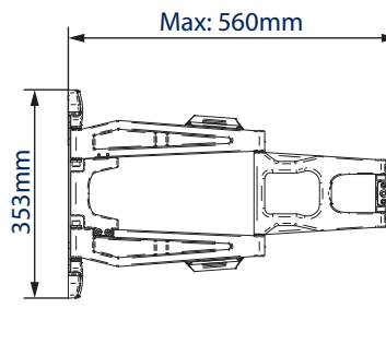
ZIJAANZICHT MAXIMALE UITREKKING
