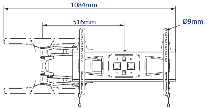
VOORAANZICHT MET DE ARM GESTREKT NAAR DE ZIJKANT
