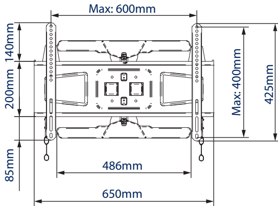
VOORAANZICHT MAXIMALE UITREKKING
