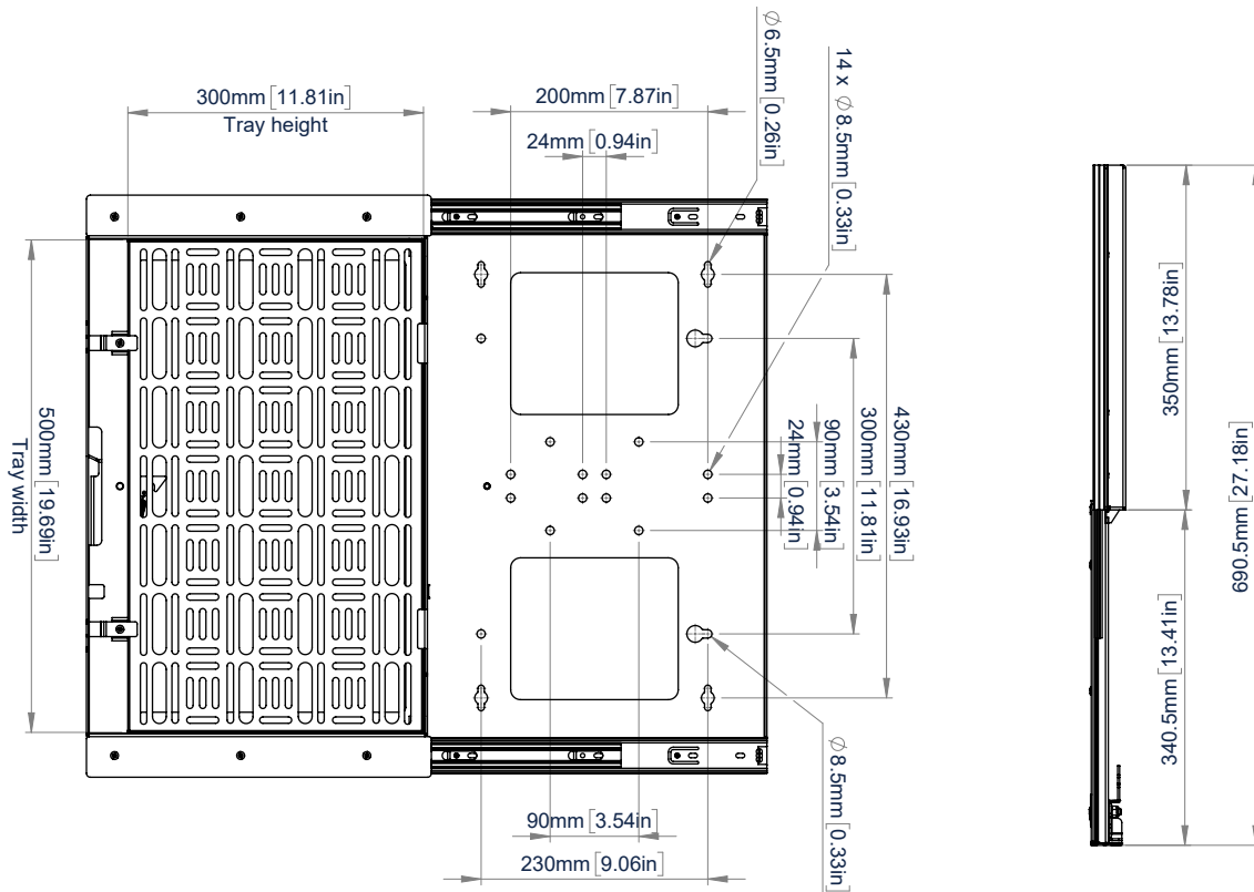
VOORAANZICHT OPEN
