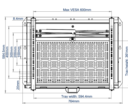
VOORAANZICHT
