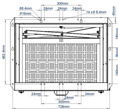
ACHTERKANT
