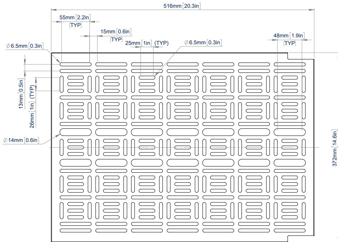
BOVENAANZICHT
