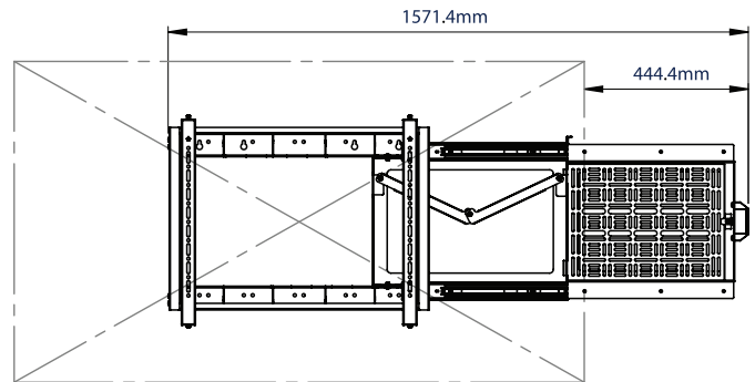
46" SCHERM OPEN
