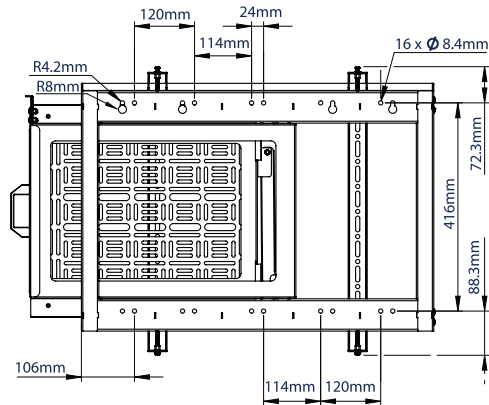
ACHTERKANT
