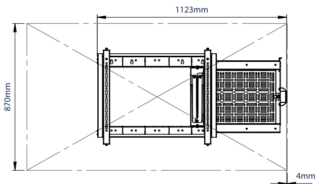
75" SCHERM GESLOTEN
