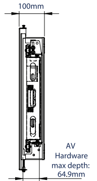
ZIJAANZICHT
