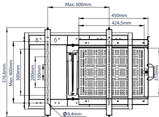
VOORAANZICHT
