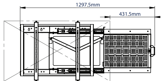
46" SCHERM OPEN
