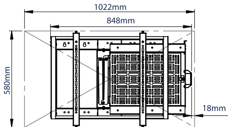
46" SCHERM GESLOTEN
