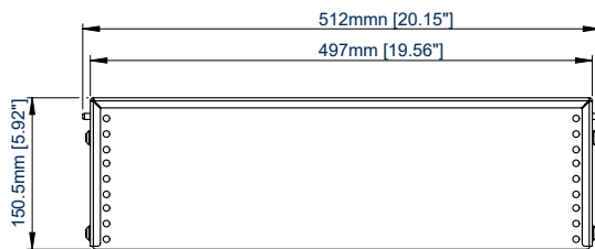
BOVENAANZICHT
