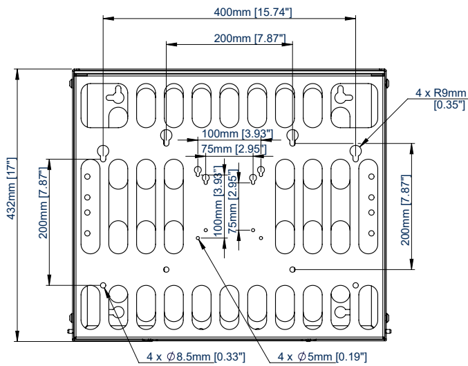
VOORAANZICHT
