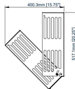
ZIJZICHT
