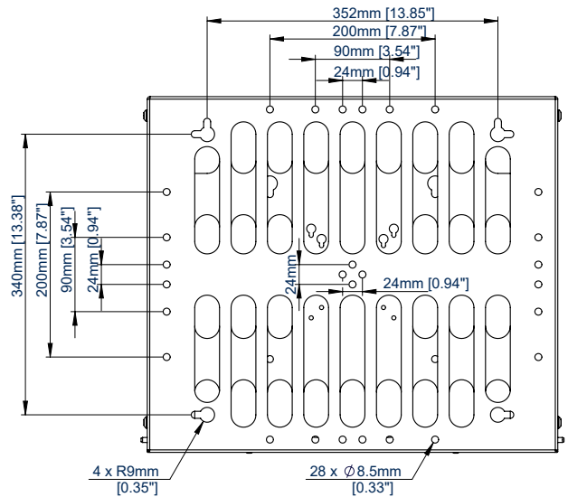
ACHTERAANZICHT
